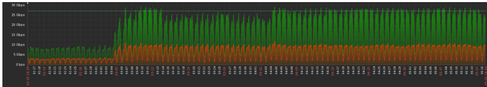
Gráfico da CDN-A durante rompimento de fibra óptica submarina em Salvador em março de 2023
